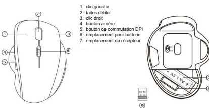
Vue dessus
